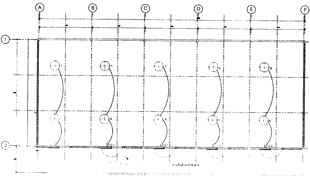
แปลนระบบทึดลมโครงห้องปฏิบัติการวิทยาศาสตร์ วพ.ภวศ.พ. SCALE 1:125
