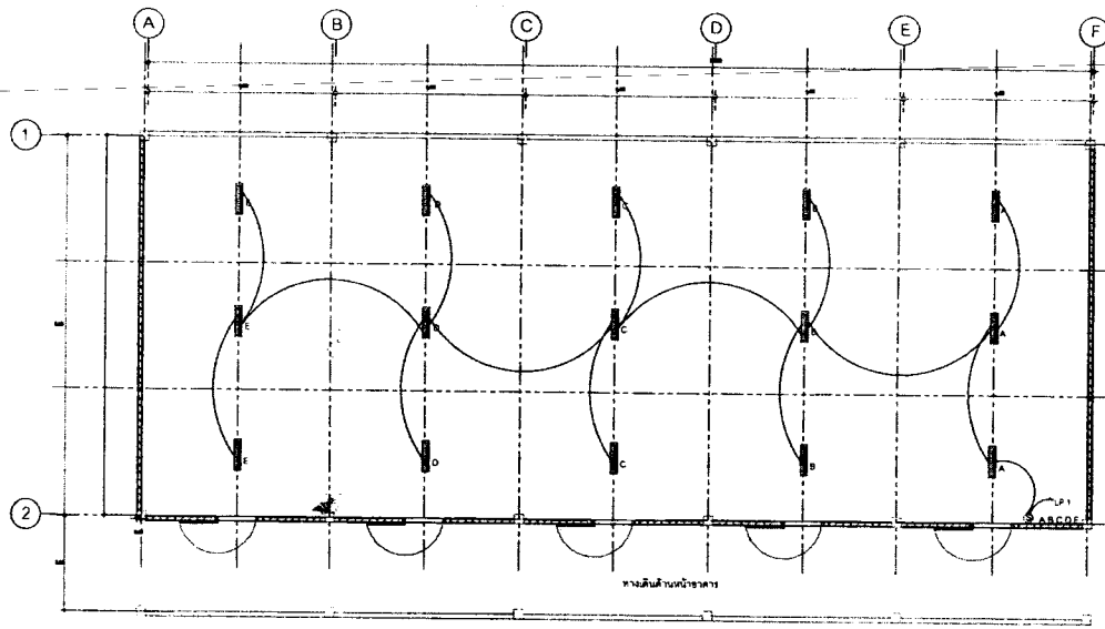
แปลนระบบไฟฟ้าแสงสว่างห้องปฏิบัติการวิทยาศาสตร์ วพ.ภวศ.พ. SCALE 1:125
