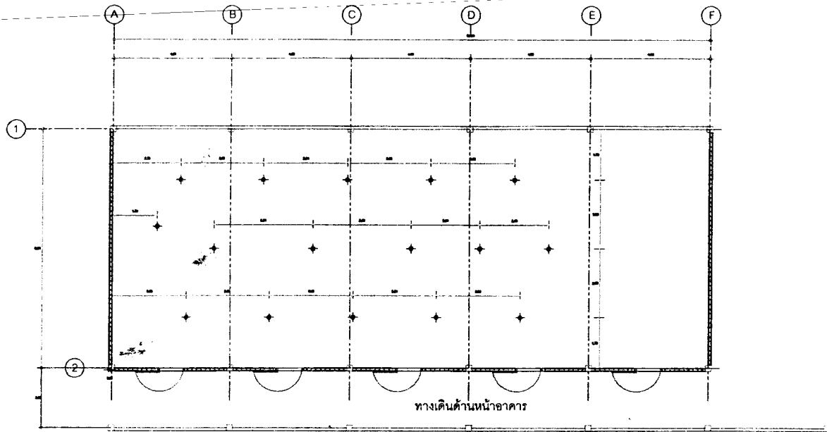
แปลนตำแหน่งท่อระบายน้ำทิ้ง SCALE 1:125
