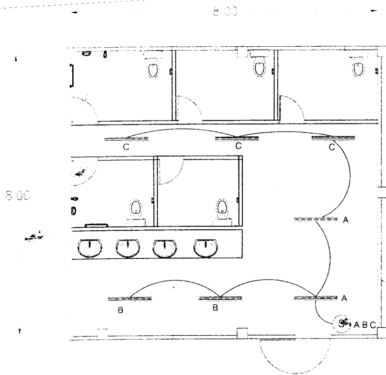
แบบขยายห้องน้ำ ชั้น 2
