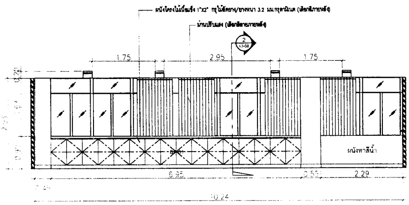
A ELEVATION 1:50
