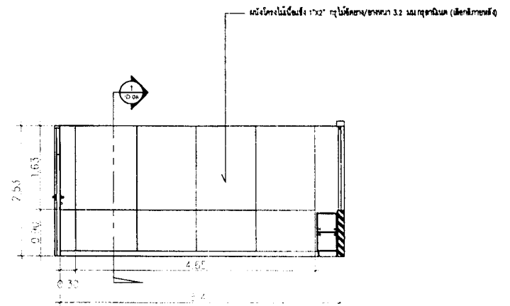
B ELEVATION 1:50
