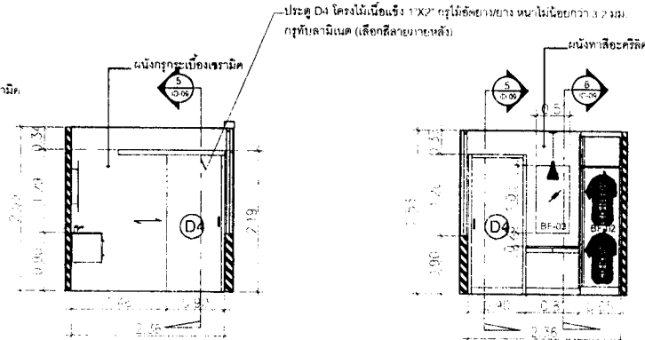
H ELEVATION 1:50 ID-06
