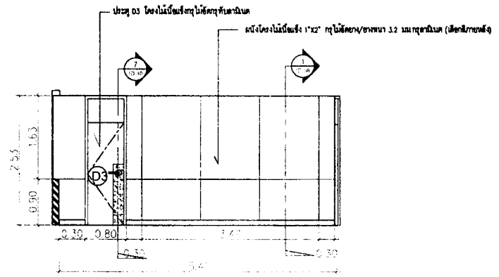
D ELEVATION 1:50
