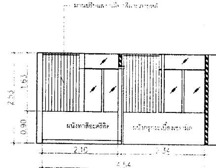
F ELEVATION 1:50 ID-04
