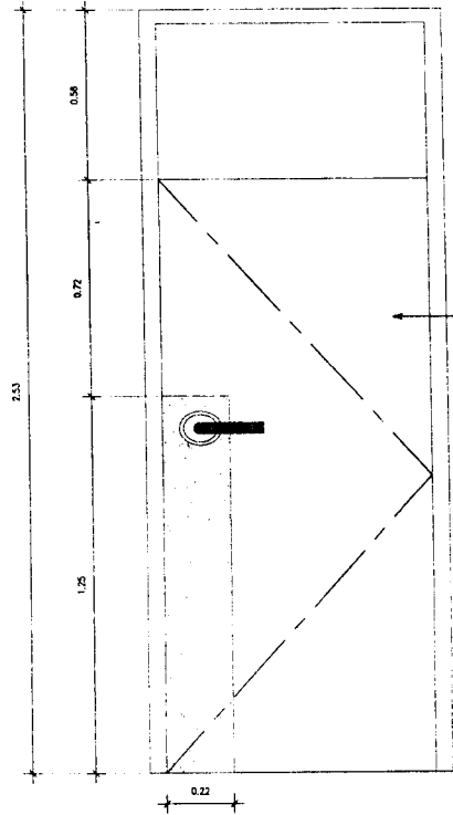
7 ELEVATION D-10 DOOR
